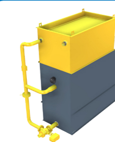
Batteria antifumana
